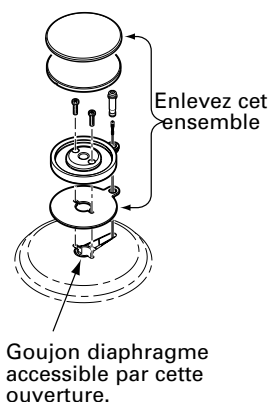
Capuchon de brûleur
