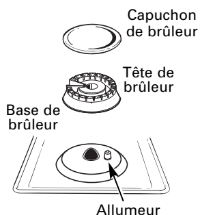
Brûleur de 18000 BTU (sur certains modèles)
