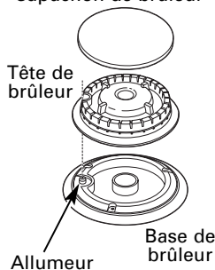
Brûleur de 18000 BTU (sur certains modèles)
