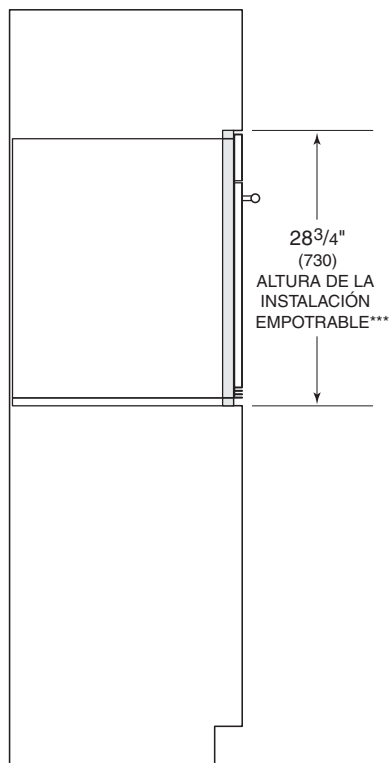
VISTA LATERAL
