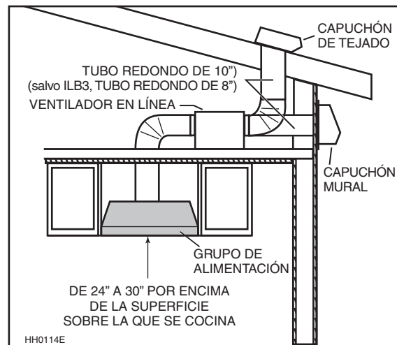
INSTALACIÓN HABITUAL DE LOS TUBOS CON UN VENTILADOR EN LÍNEA MODELO ILB3, ILB6, ILB9 O ILB11 DE LA SERIE CP47E (UBICACIÓN DEL VENTILADOR SÓLO A MODO DE EJEMPLO)
