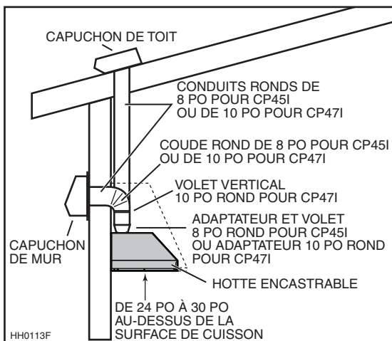
INSTALLATION TYPE CP45I MODÈLE (VENTILATEUR INTERNE SIMPLE) OU CP47I (VENTILATEUR INTERNE DOUBLE)
