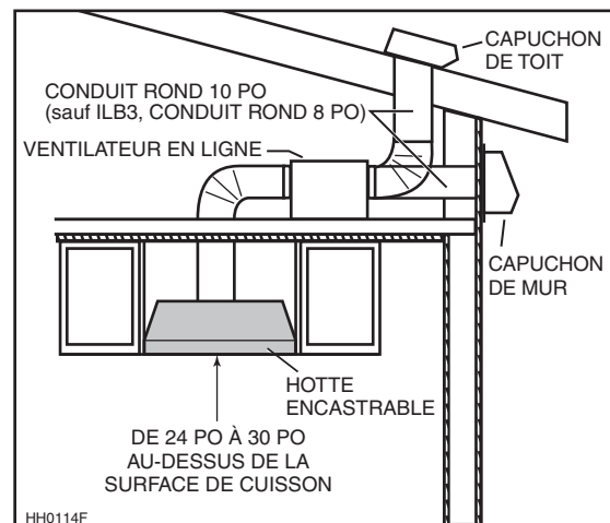
INSTALLATION TYPE VENTILATEUR EN LIGNE CP47E MODÈLE ILB3, ILB6, ILB9 ou ILB11 L'EMPLACEMENT DU VENTILATEUR EST ILLUSTRÉ À TITRE DE RÉFÉRENCE SEULEMENT
