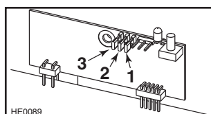
PUENTES DE LA TARJETA DE CIRCUITOS LINKLOGIC
