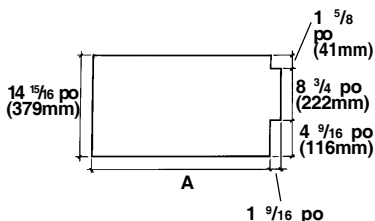
DÉCOUPER UN TROU DANS LA BASE DE L'ARMOIRE
