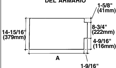
HACER LA ABERTURA EN LA BASE DEL ARMARIO
