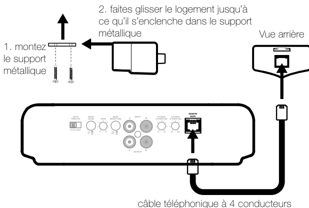
câble téléphonique à 4 conducteurs
