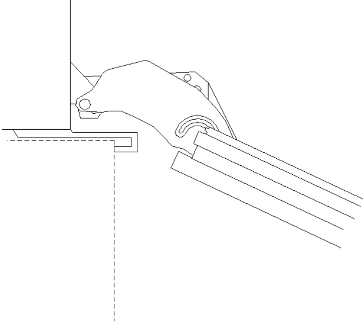
Door Swing
