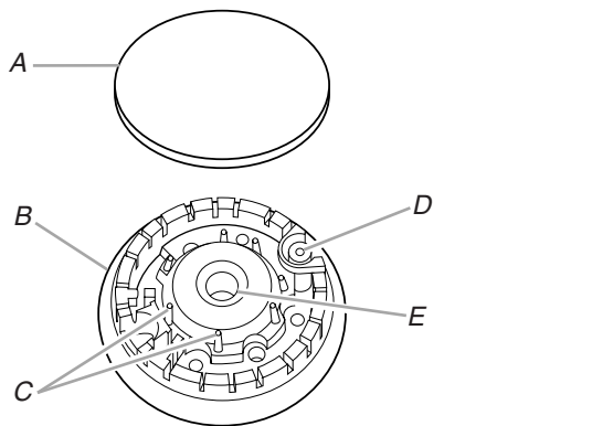
A. Chapeau de brûleur B. Base du brûleur C. Tiges d'alignement D. Dispositif d'allumage E. Ouverture du tube d'arrivée de gaz
