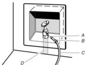
A. Ampoule B. Écrou C. Tuyau en cuivre ou en polyéthylène réticulé (vers le réfrigérateur) D. Conduite d'alimentation du domicile (1/2 po minimum)
