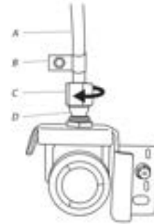
A. Tuyau en cuivre ou en polyéthylène réticulé B. Collier en « P » C. Écrou de compression D. Virole de compression
