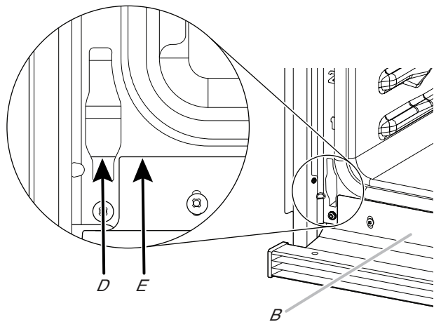
A. Marco del horno B. Lengüeta de la moldura C. Tornillo n.º 8-18 x 3/8" (9,5 mm) D. Borde del receptor de bisagra E. Parte superior de la lengüeta de la moldura de ventilación inferior
