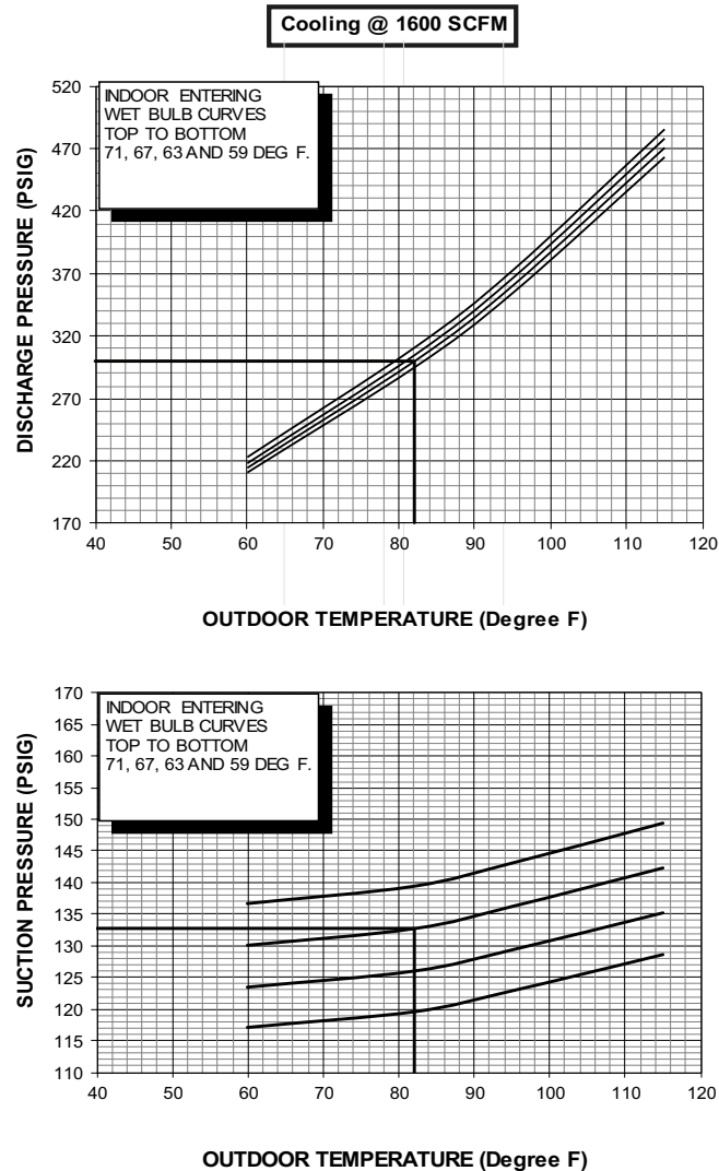
Figure 23. 5 Ton AC (060 Models)
