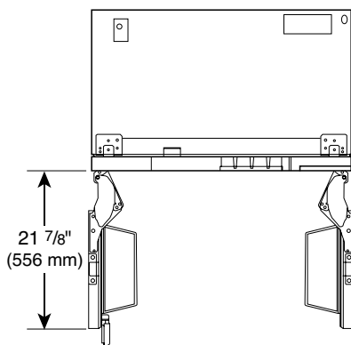
VUE DE DESSUS PORTE OUVERTE 90°
