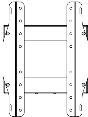
VESA 200 X 100
