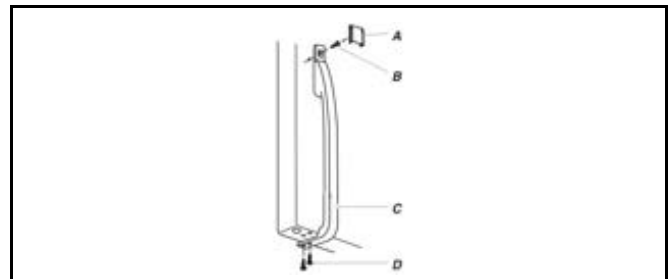
A. Cache-vis C. Poignée du congélateur B. Vis de poignée D. Vis de poignée à tête plate
