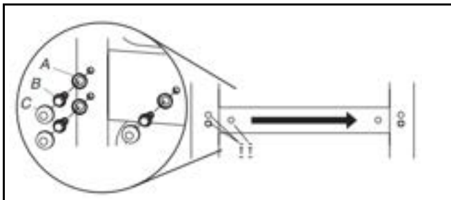
A. Rondelles de chapeaux bombés C. Chapeaux bombés B. Vis de charnière à tête hexagonale
