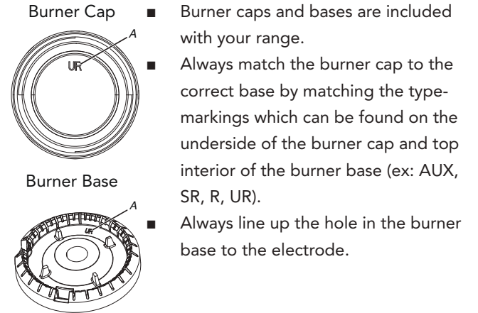
A. Burner Cap Symbol
