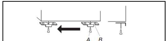
A. Door Stop Screw B. Door Stop
