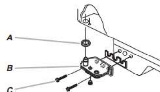
C. Vis de charnière à tête hexagonale de 5/16 po
