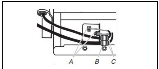
A. Wiring plugs C. Grommets B. Wiring clip
