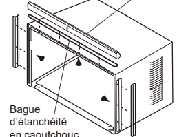
FIG.8 Rail d'angle supérieur
