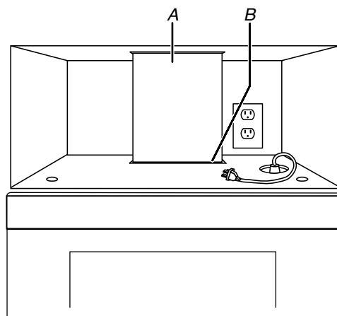
A. Système d'extraction B. Clapet (sous le conduit d'évacuation) – compact
