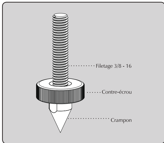
Le crampon ETC.
