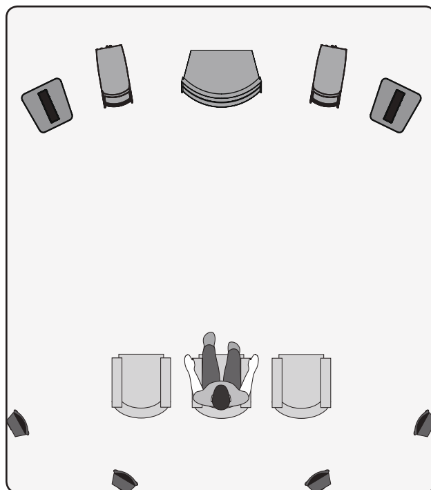
Enceintes électrostatiques MartinLogan en tant que canaux avant, canal central et canaux ambiophoniques (effets) arrière et latéraux. Caissons de sous-graves MartinLogan en tant que canal LFE (effets).
