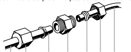
A. Tube vers le réfrigérateur B. Écrou (fourni) C. Renflement D. Raccord (fourni) E. Virole (à acheter) F. Écrou (à acheter) G. Canalisation d'eau du domicile
