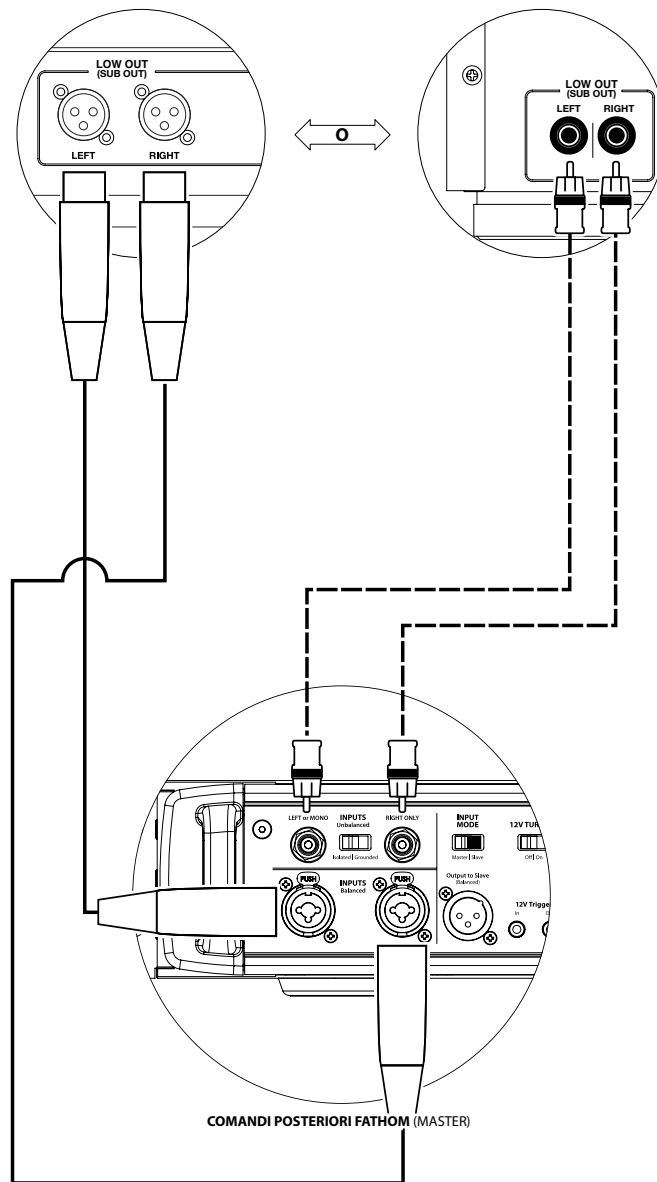
CROSSOVER ATTIVO STEREO (USCITE BILANCIATE)
