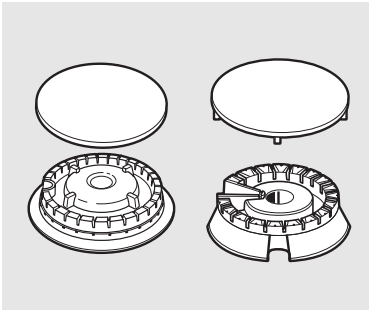
Cabezales y tapas de quemadores de superficie
