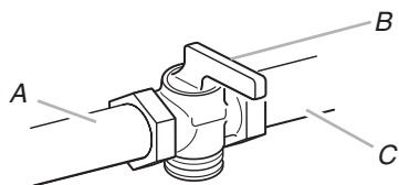
A. Vers la cuisinière B. Robinet d'arrêt manuel - manette à la position de fermeture C. Canalisations de gaz
