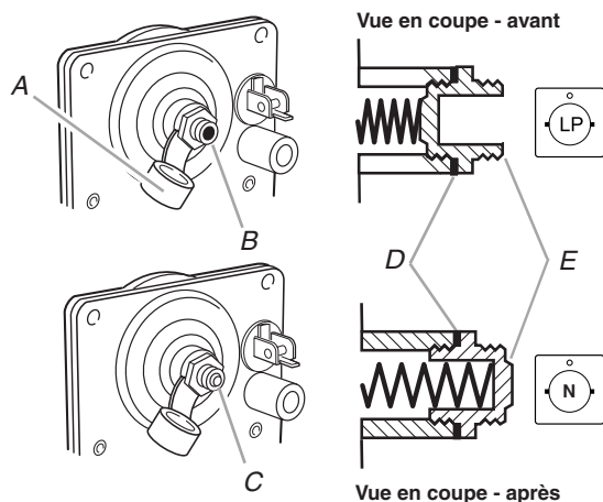
A. Couvercle de plastique B. Capuchon du détendeur; extrémité ouverte vers l'extérieur C. Capuchon du détendeur, extrémité borgne vers l'extérieur D. Joint E. Capuchon du détendeur
