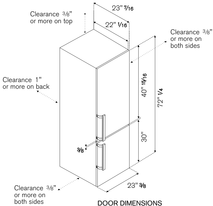
DOOR DIMENSIONS
