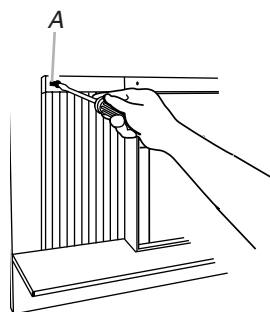
A. Tornillo de cabeza redonda #10 x \frac{3}{4} "
