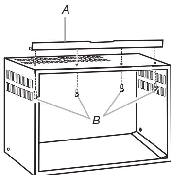
A. Canal superior B. Tornillos de cabeza de arandela Phillips de roscar #10 x \frac{3}{8} "
